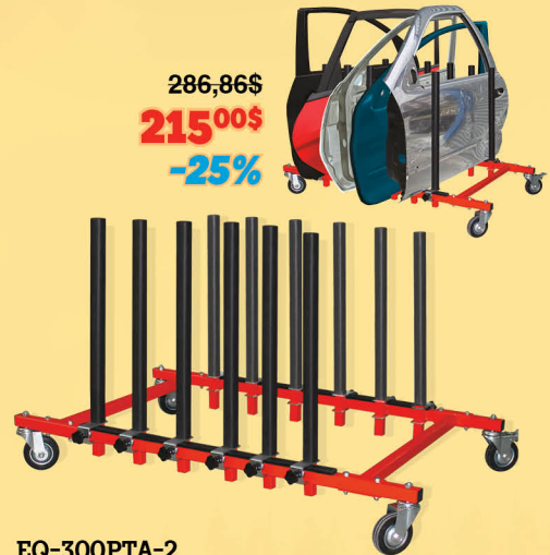
EQ-300PTA-2 Mobile Rack for panels, doors, hoods and windshields Étagère mobile pour panneaux, portes, capots et pare-brises
